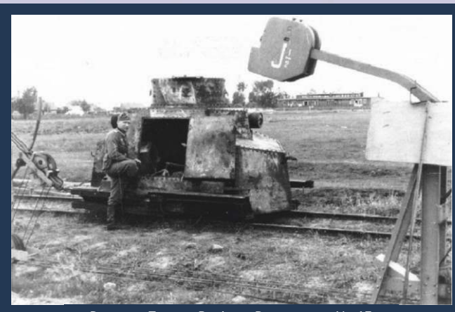
Drezyna Tatra z Pociągu Pancernego Nr 13.
